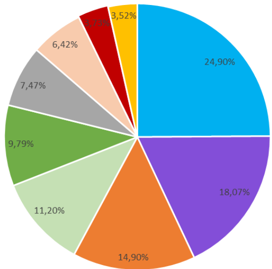
Индикаторы ботнетов
