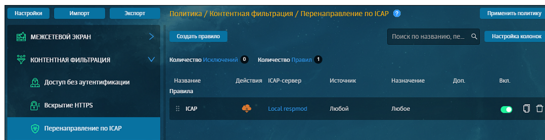
Рис. 6.32. Слой правил политики «Перенаправление по ICAP»
