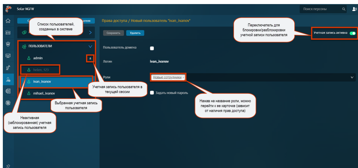
Рис. 8.11. Раздел «Пользователи > Пользователи»
