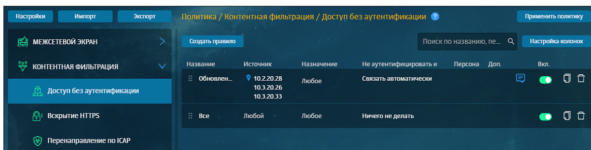
Рис. 6.30. Слой правил политики «Доступ без аутентификации»
