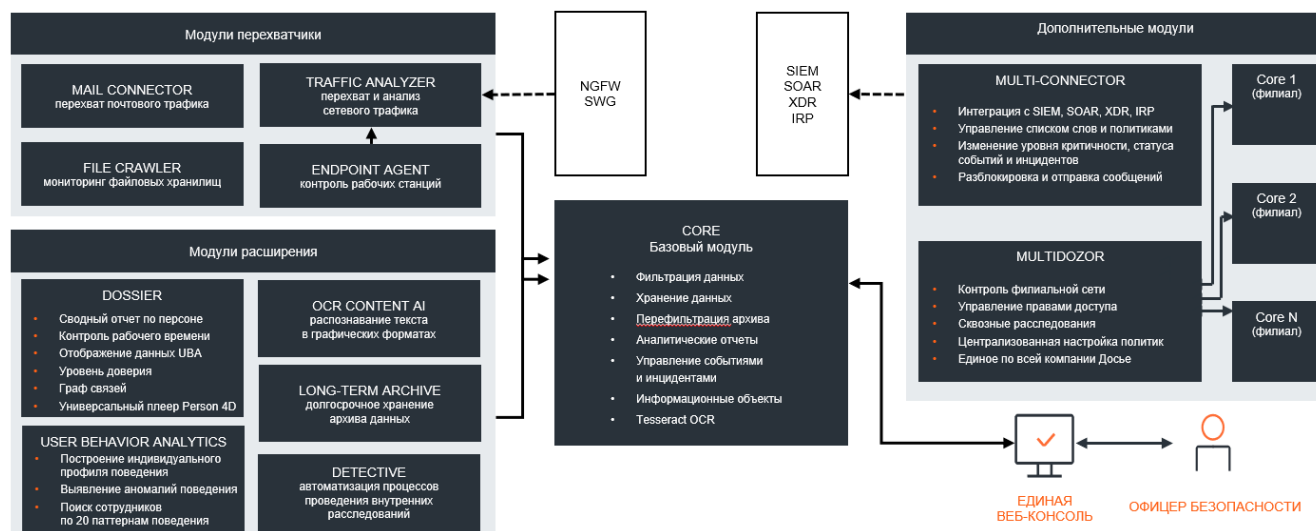
Рисунок 71. Концептуальная архитектура Solar Dozor
