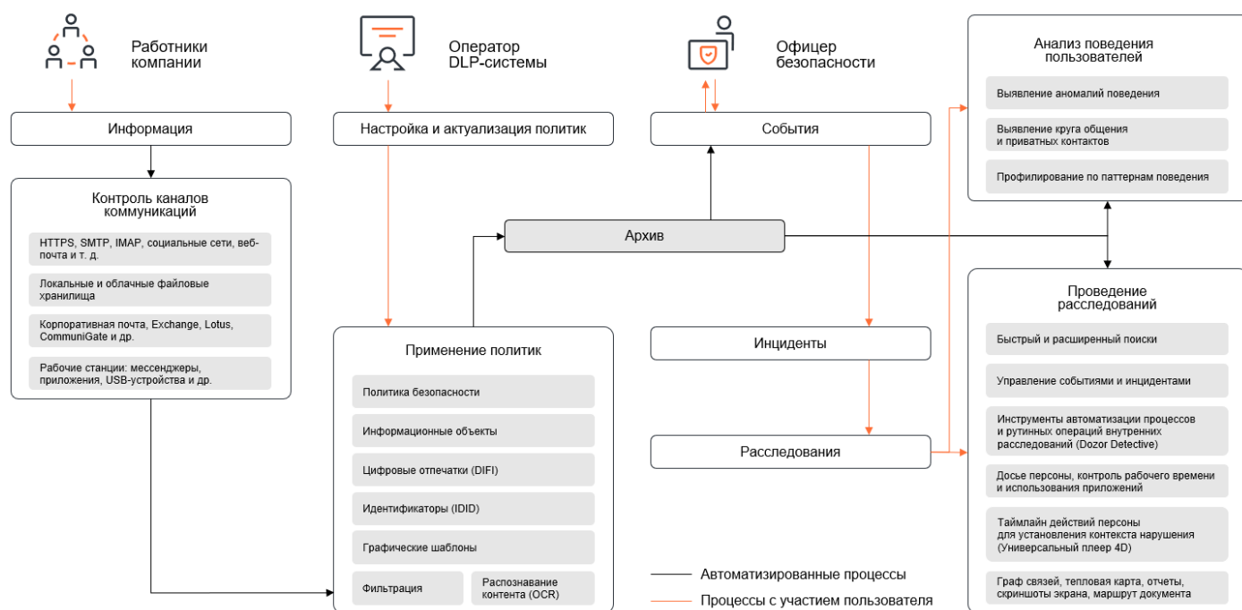
Рисунок 1. Концептуальная схема работы Solar Dozor
