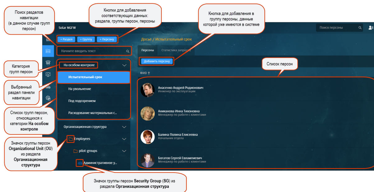
Рис. 5.1. Раздел «Досье»
