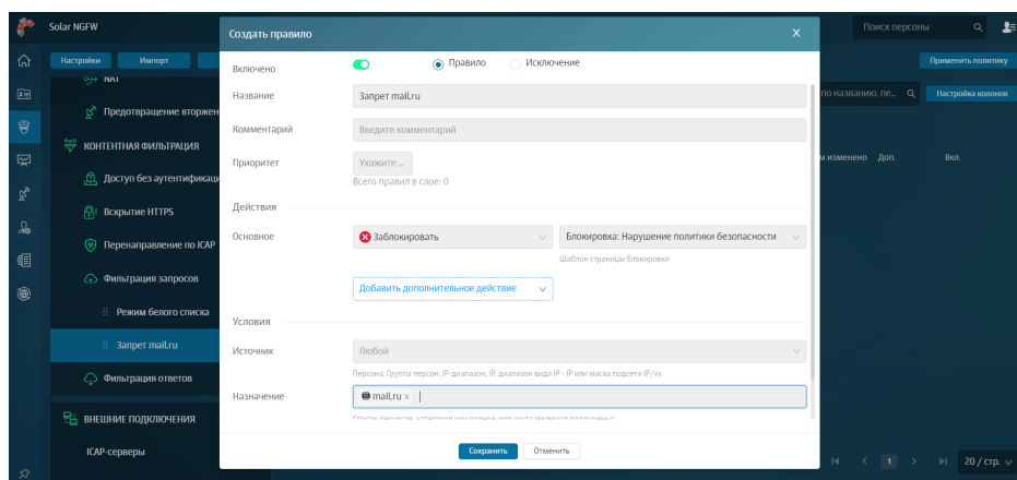
Рис. 6.78. Формирование правила
