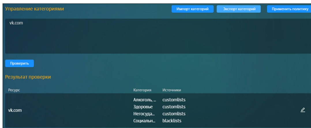
Рис. 6.91. Проверка категории
