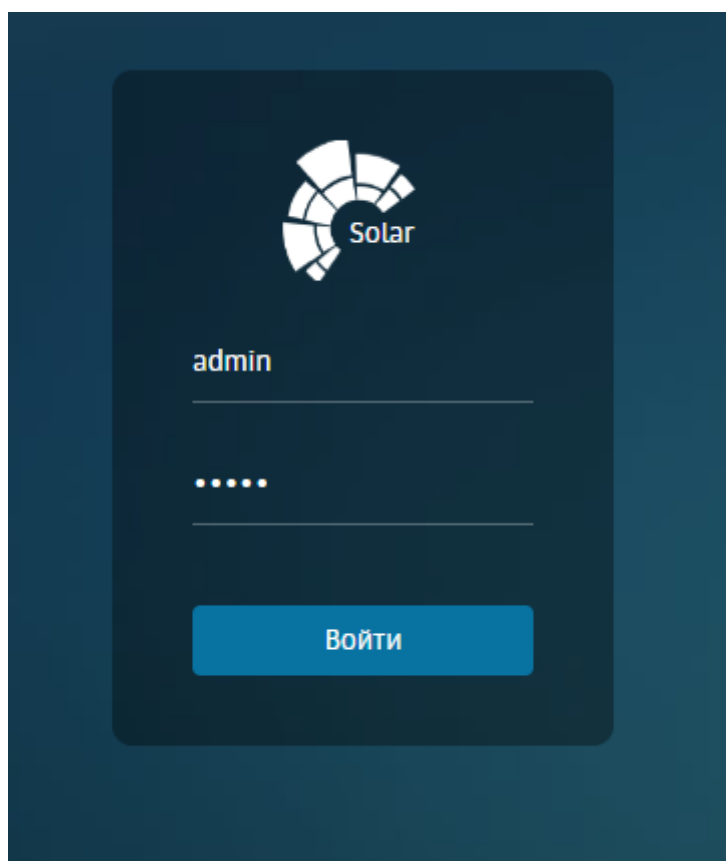
Рис. 3.3. Авторизация
