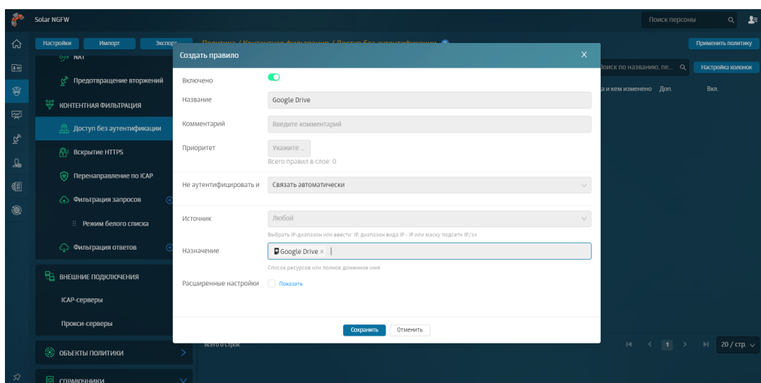
Рис. 6.69. Формирование правила
