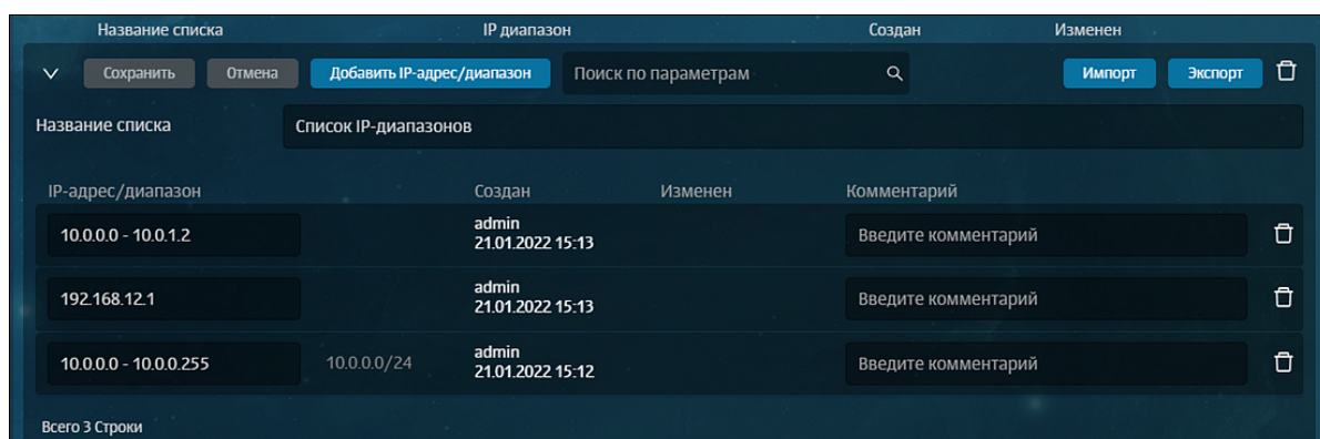
Рис. 6.37. Форматы IP-диапазонов
