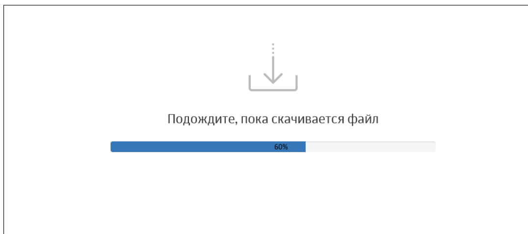
Рис. 6.87. Статус загрузки
