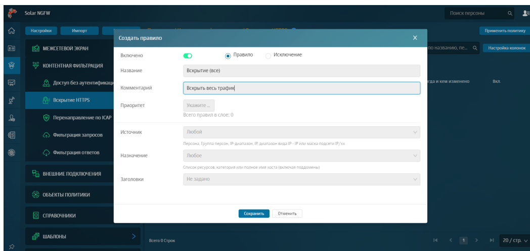
Рис. 6.70. Формирование правила
